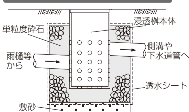
雨水浸透施設(浸透枡)の設置例
