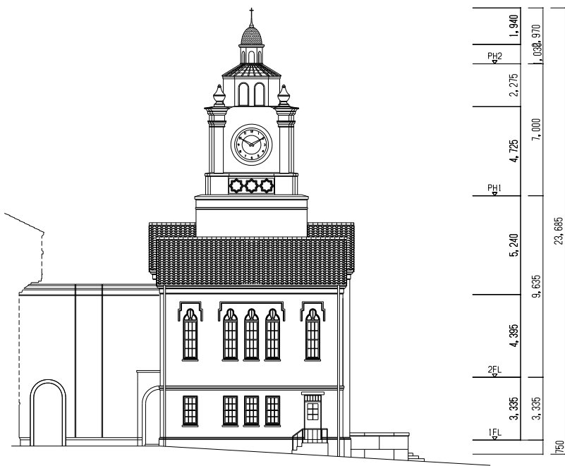
南立面図
