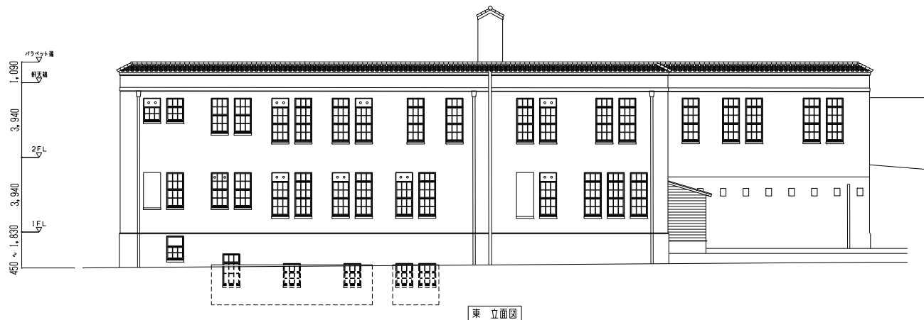
東立面図
