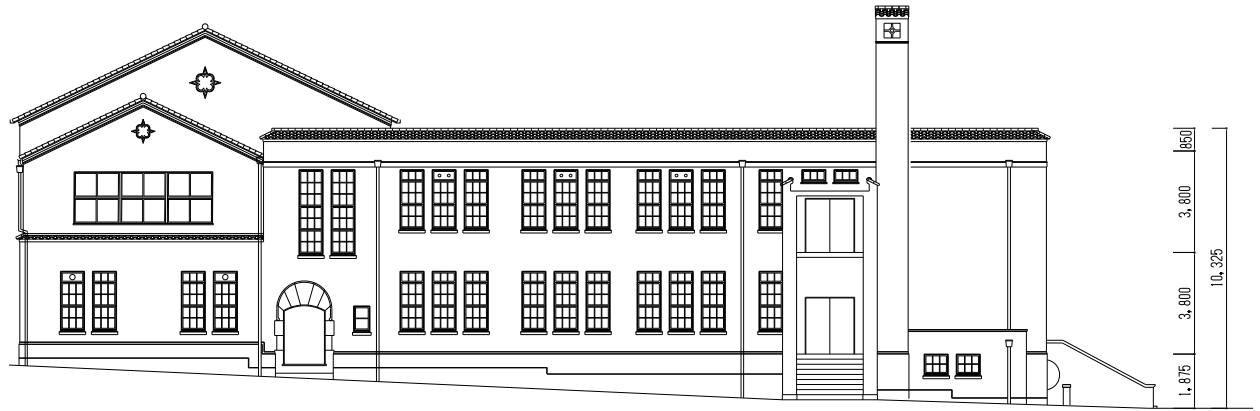
南立面図
