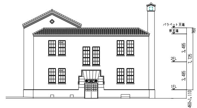
東立面図
