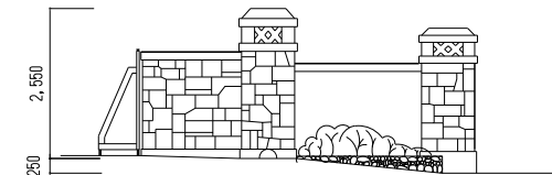
北立面図
