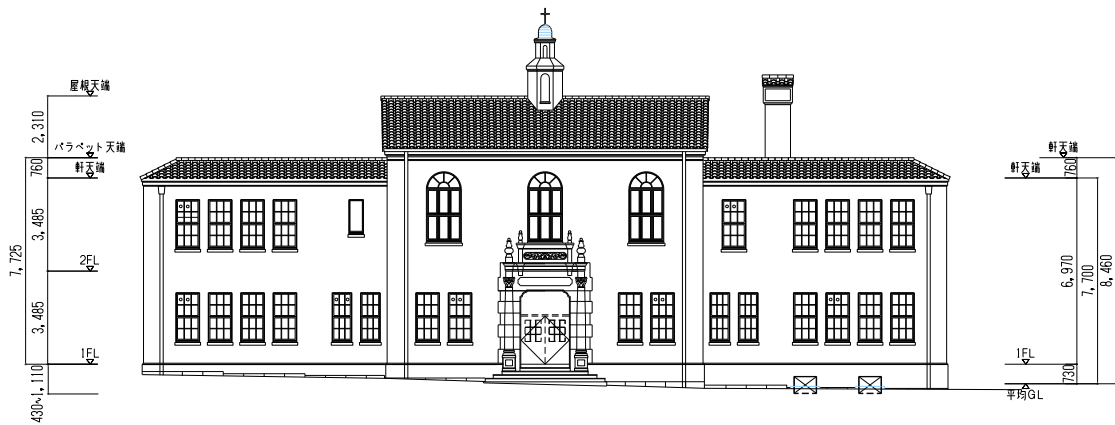
南立面図
