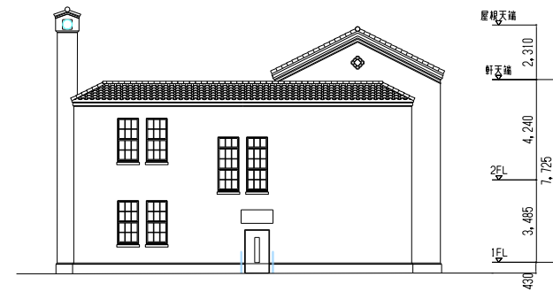
西立面図
