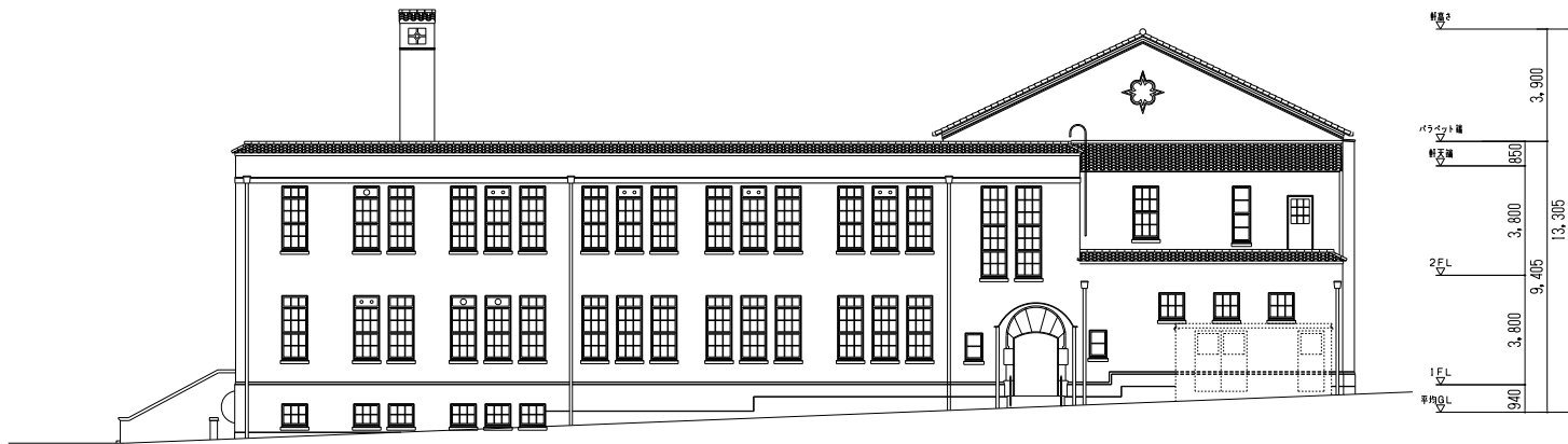
北 立面図
