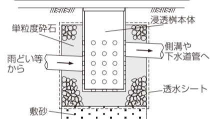
雨水浸透施設(浸透枳)の設置例
