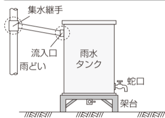
雨水貯留施設(雨水タンク)の設置例
