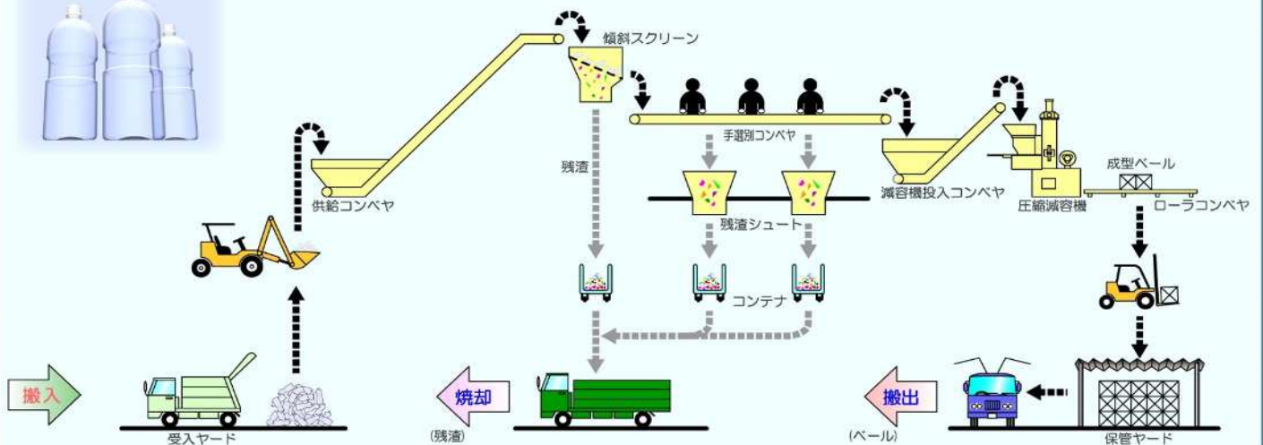
■ 処理系統図 ■
