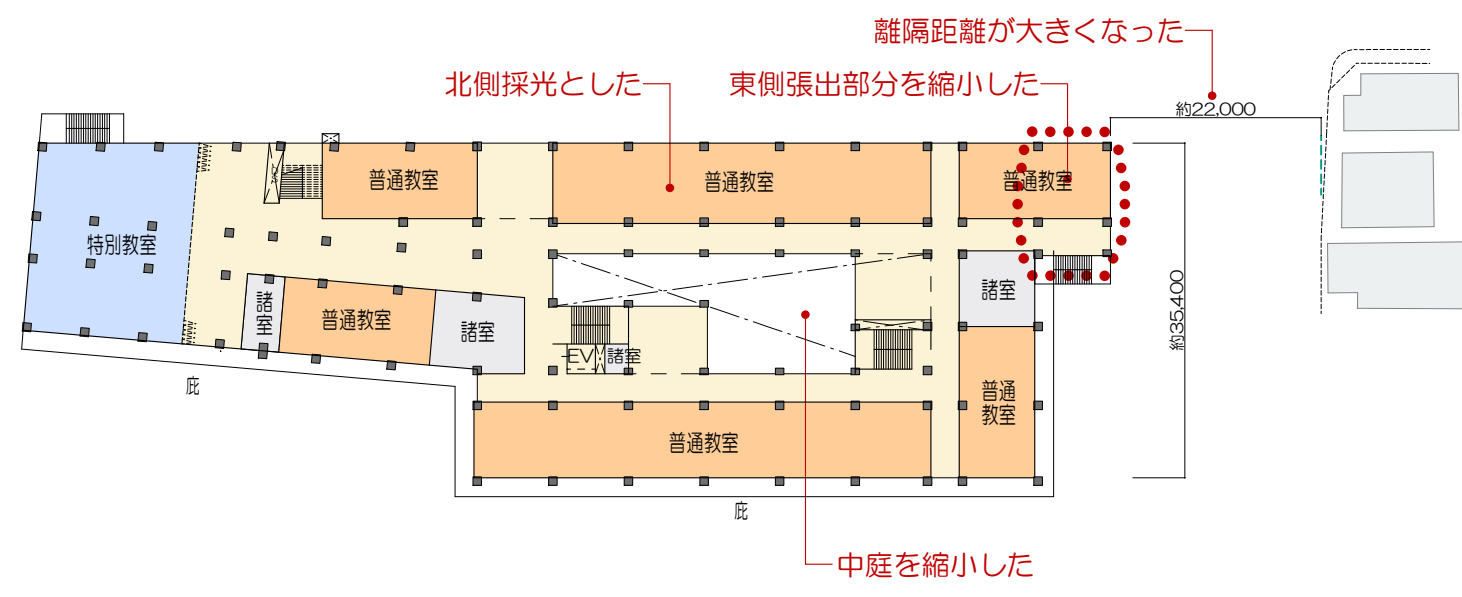
2階平面図
