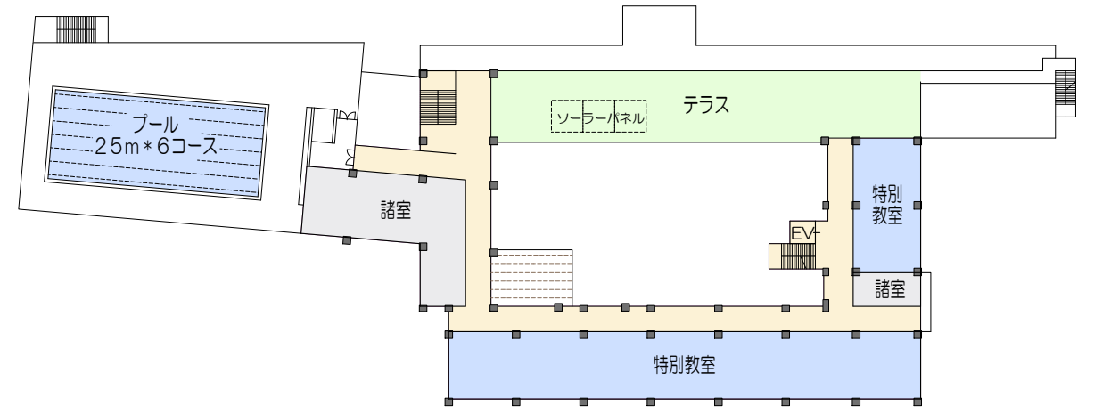
4階平面図
