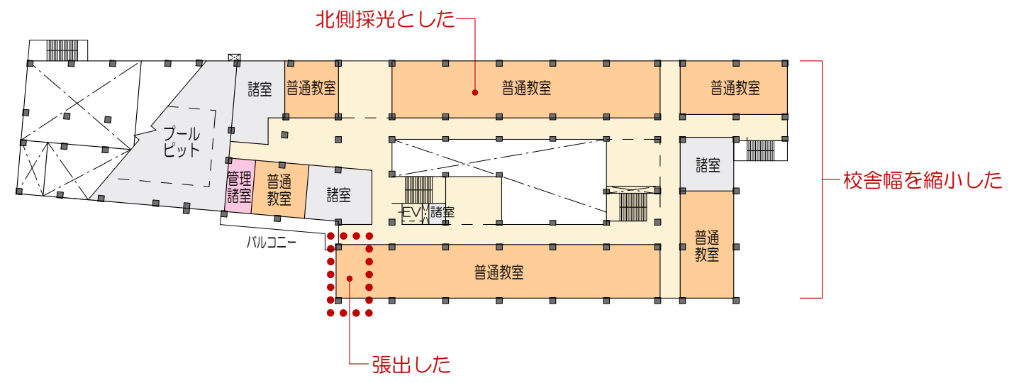
3階平面図
