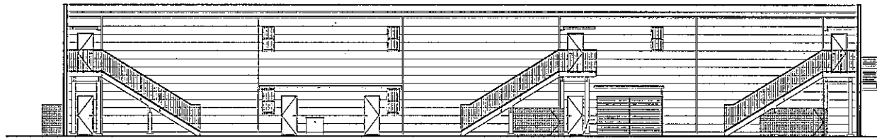
【北立面图】
